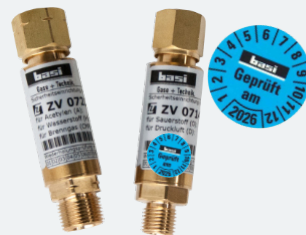
Gebrauchsstellenvorlagen (Thermomate)
